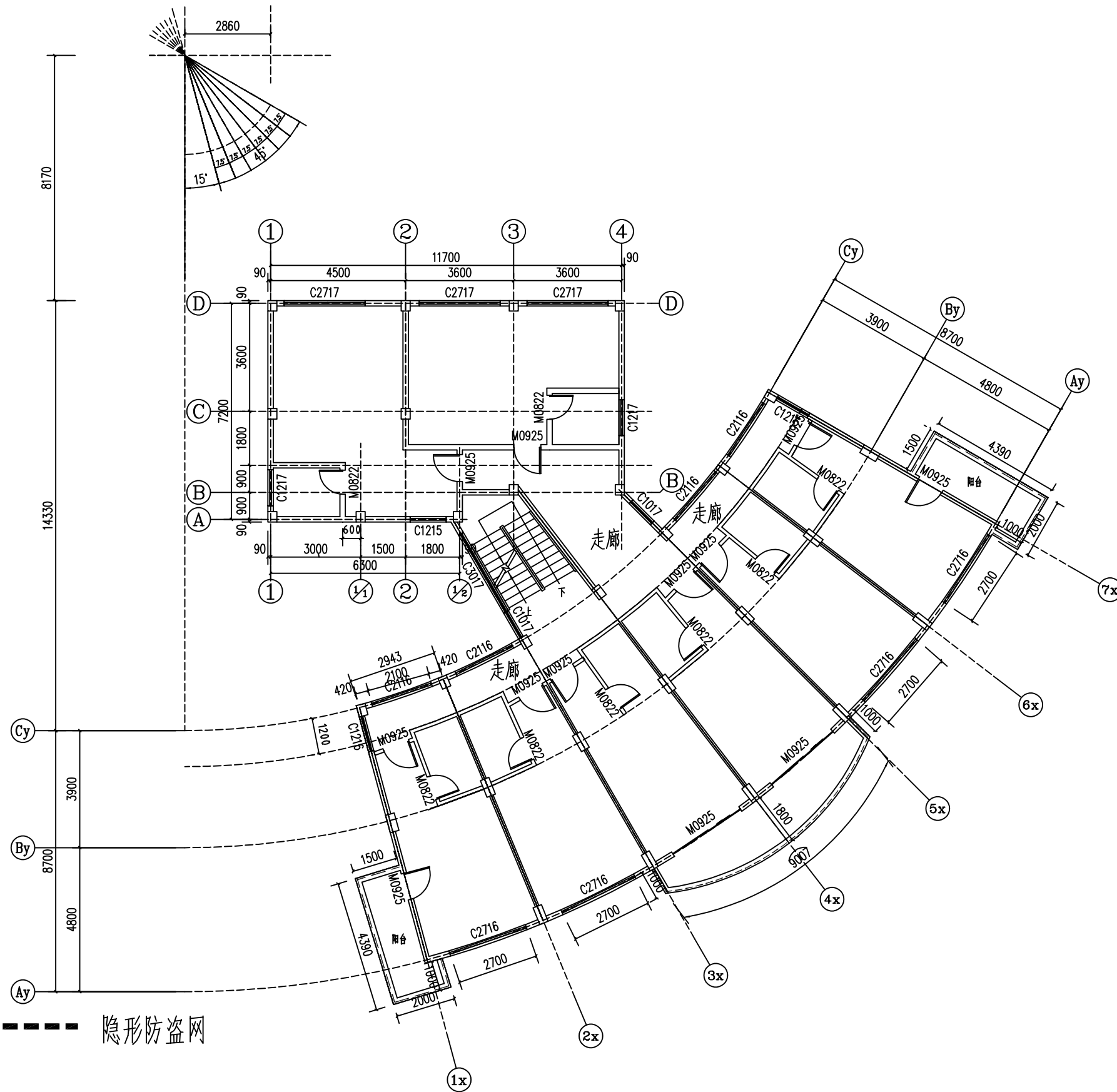
招待所5层平面布置图 1:100
