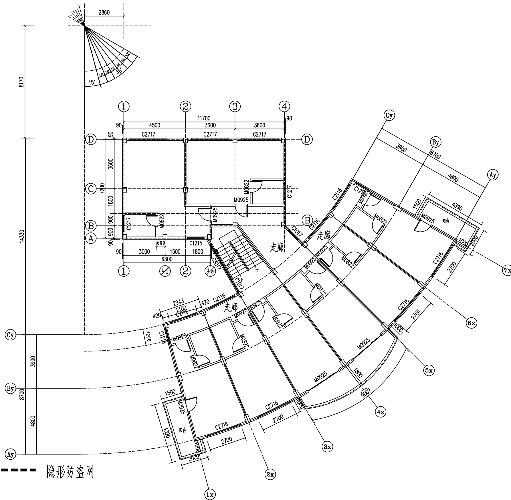
招待所4层平面布置图 1:100
