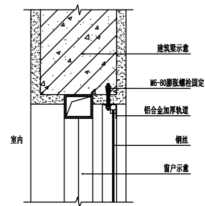
隐形防盗网/阳台罩大样 1:5
