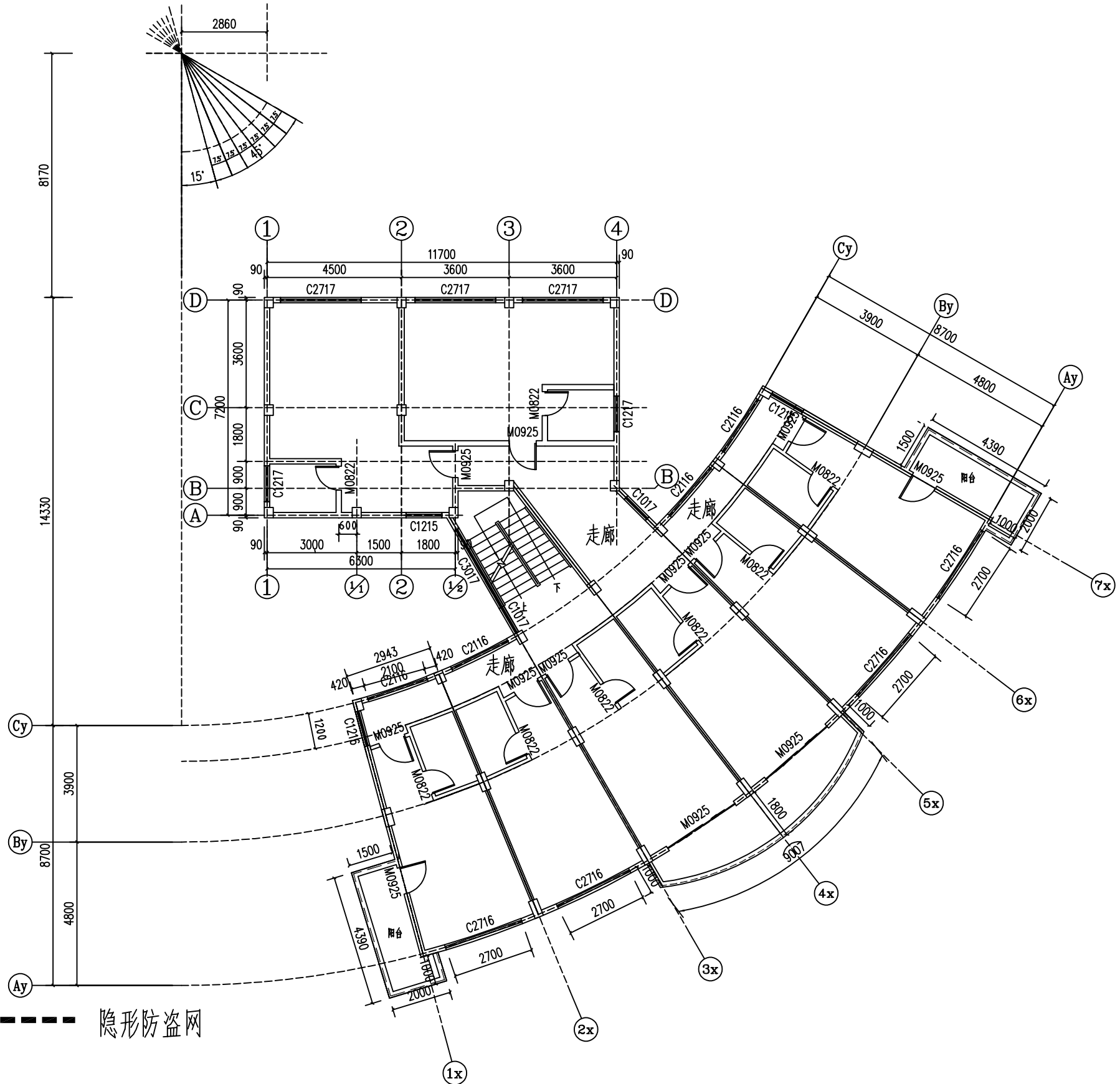
招待所2层平面布置图 1:100
