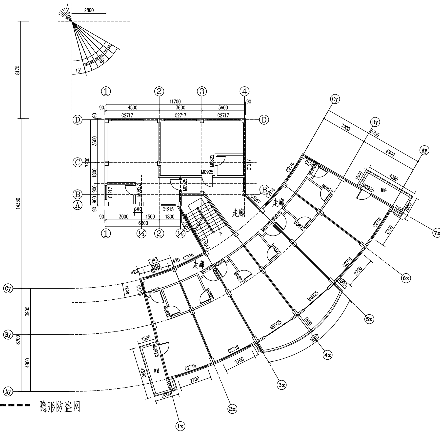
招待所3层平面布置图 1:100
